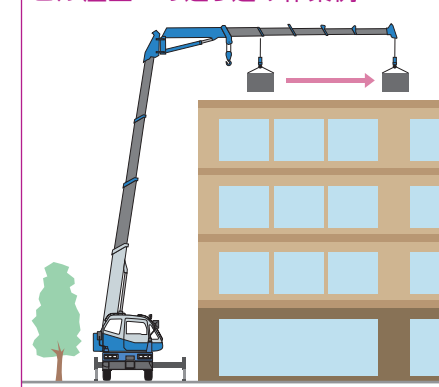
ビル屋上への送り込み作業例
